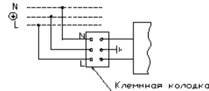
Схема.2 Схема подключения с регулируемым ЭПРА
