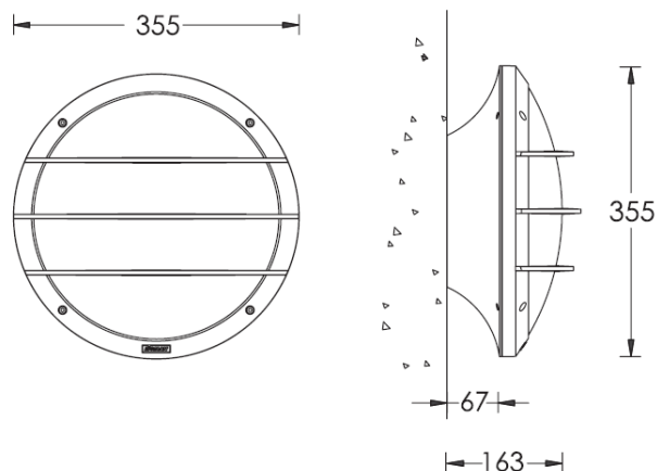
Габаритные размеры, рис.1:
