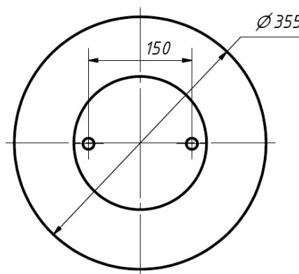
Установочные размеры, рис.2:
