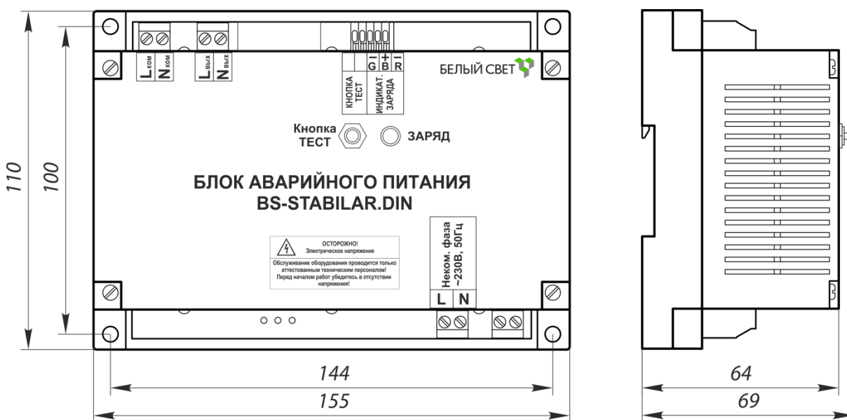
Рис. 2 Габаритный и монтажный чертеж.
