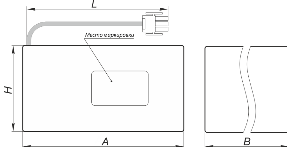
Рис. 1 Габаритный чертёж батареи
