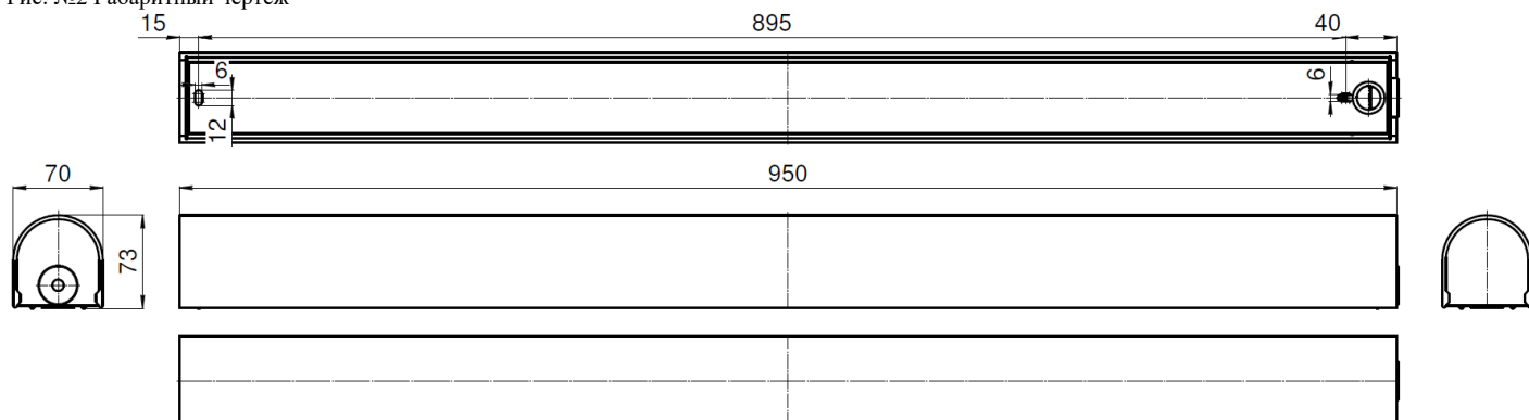
Рис. №2 Габаритный чертёж
