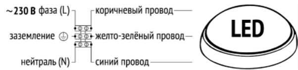
Рис.1. Схема подключения светодиодного светильника к эклектической сети 230В.
